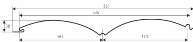
Чертеж металлического сайдинга «Бревно»
