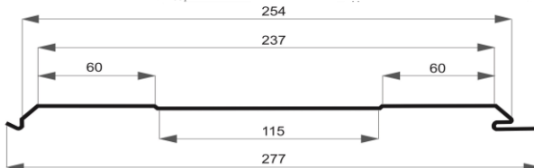
Чертеж металлического сайдинга "Доска"
